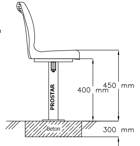
Ansicht seitlich
