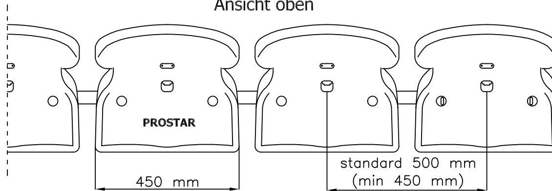
Ansicht oben
