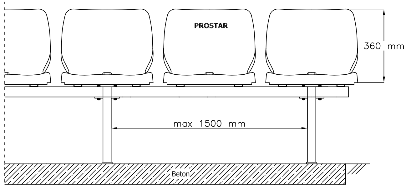
Ansicht vorn
