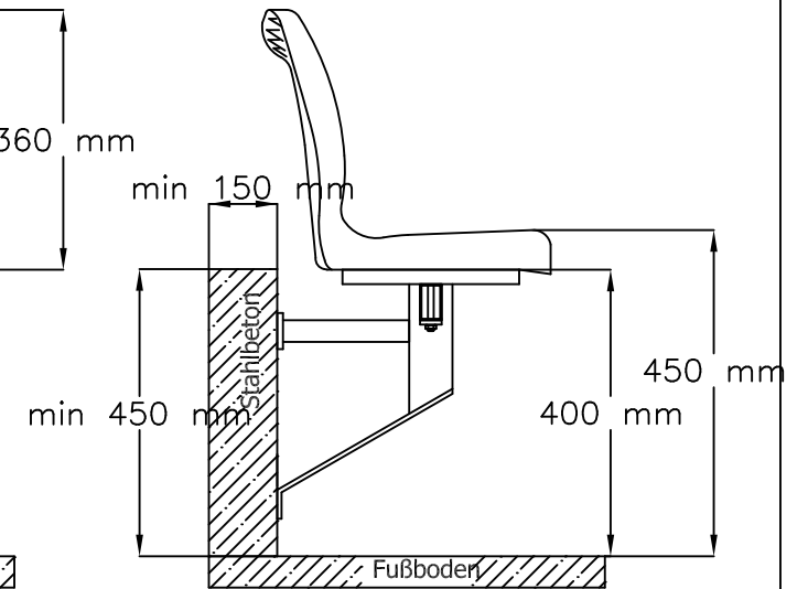
Ansicht seitlich
