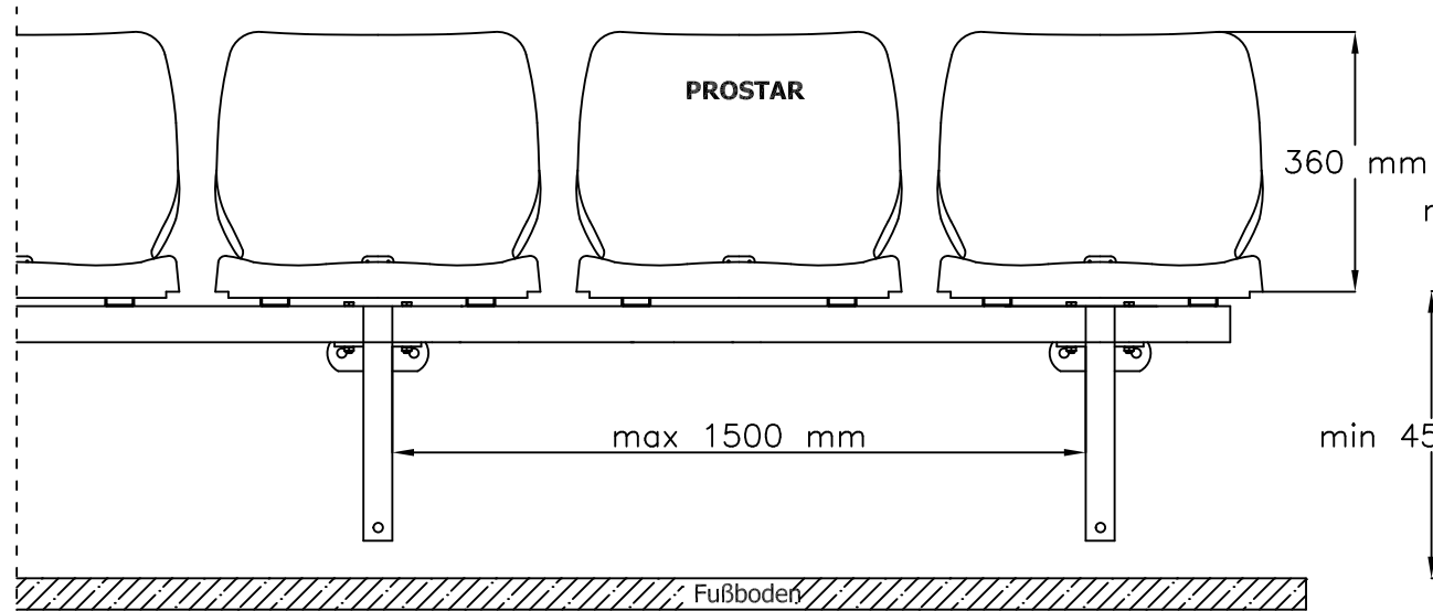
Ansicht vorn
