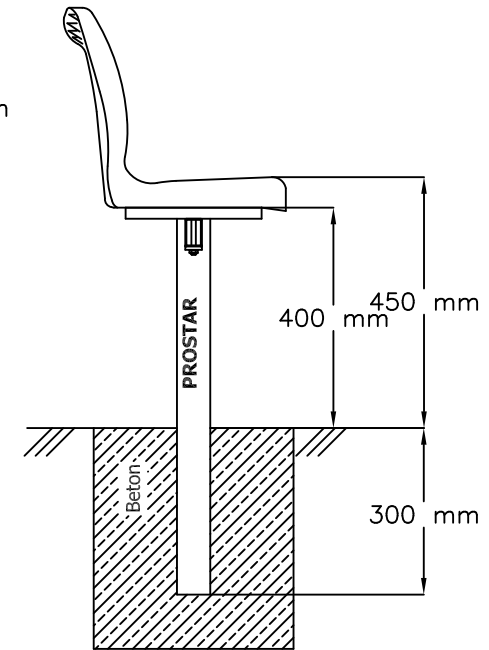
Ansicht seitlich
