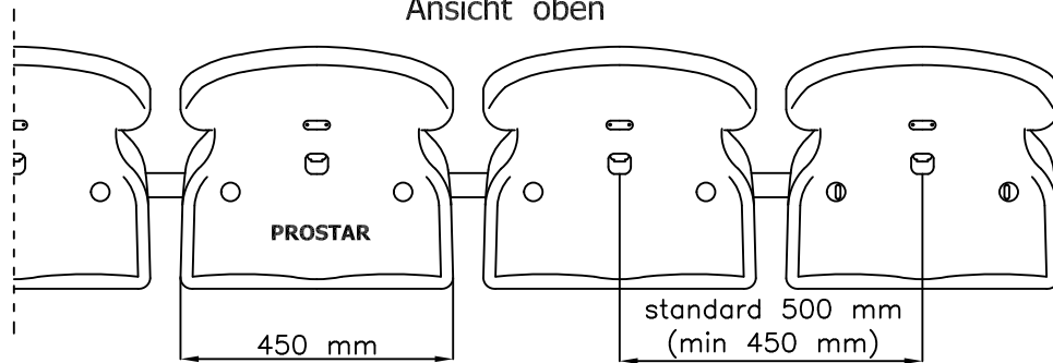
Ansicht oben
