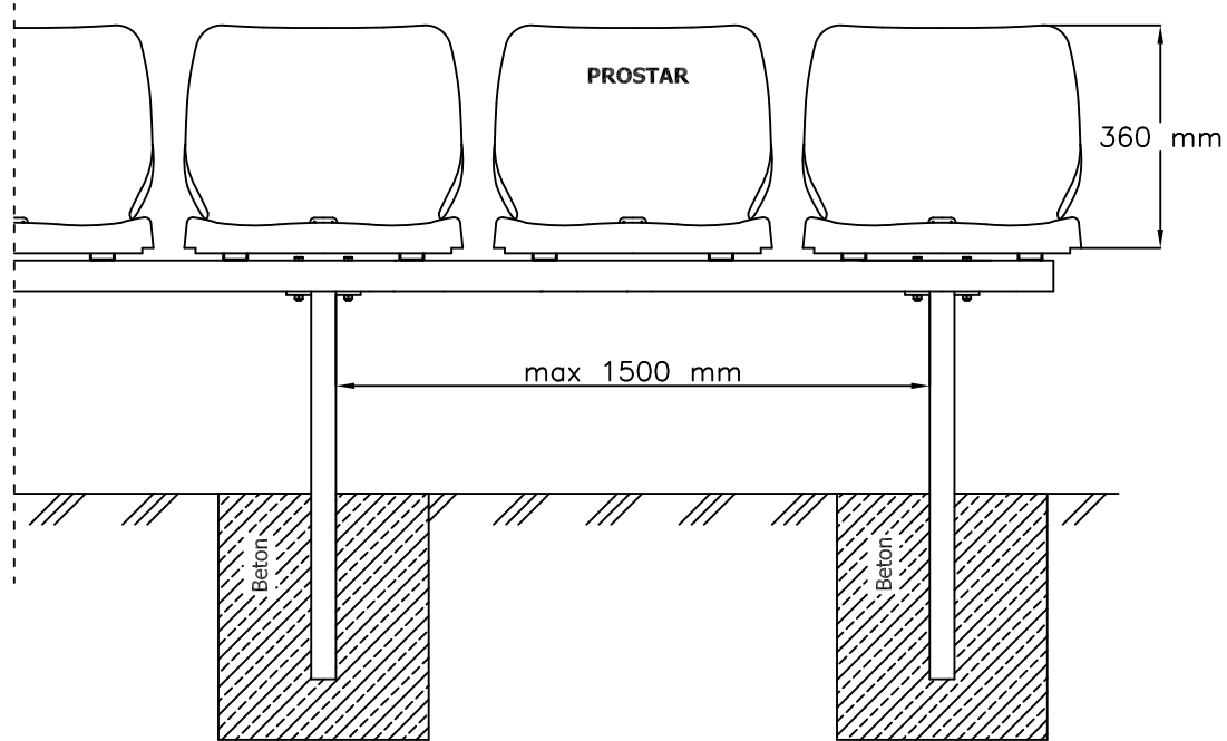
Ansicht vorn
