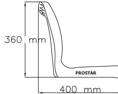
Ansicht seitlich
