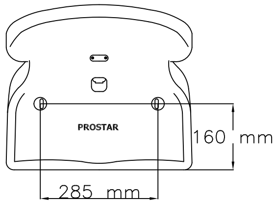
Ansicht oben
